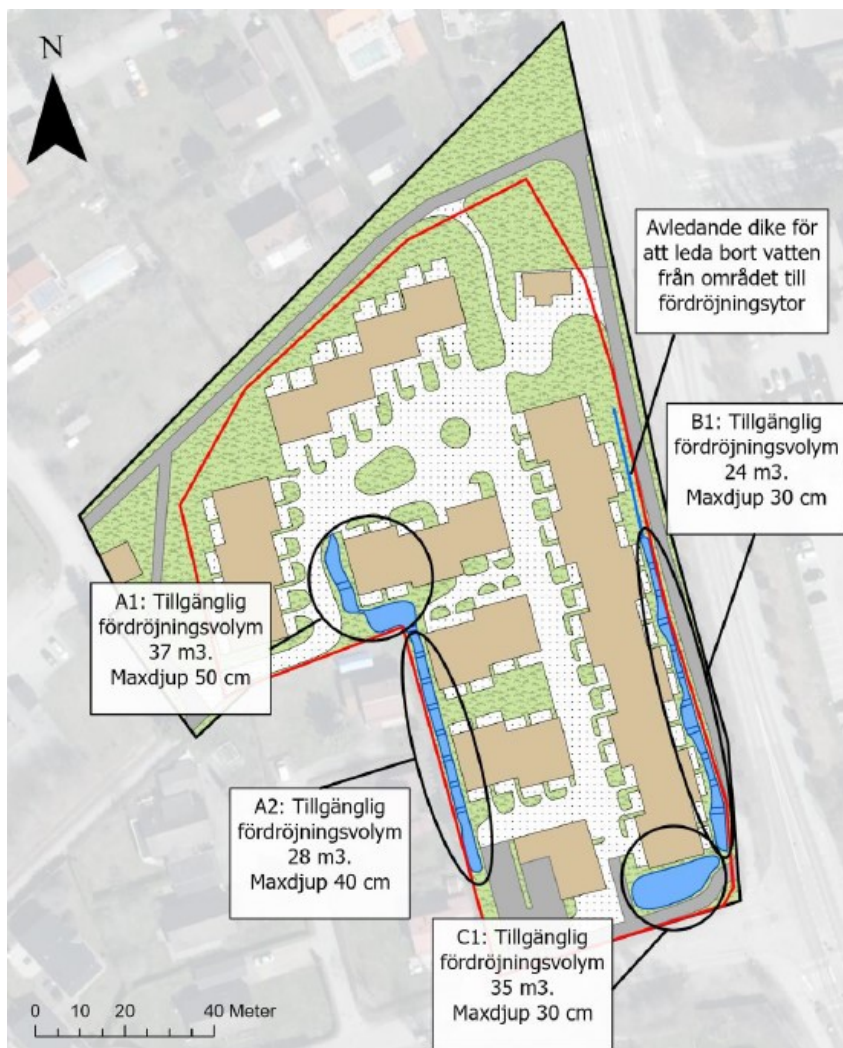
Figur 22. Principförslag för dagvattenhantering. Fastighetsgräns för Bromsen 11 är markerad med röd linje. Volym för respektive yta samt maximaldjup presenteras i figuren.
